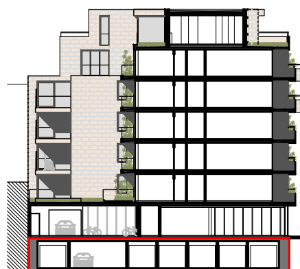
ACHTERGEVEL TOEKOMSTSTRAAT
