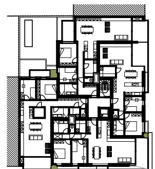
VERDIEPING +2
